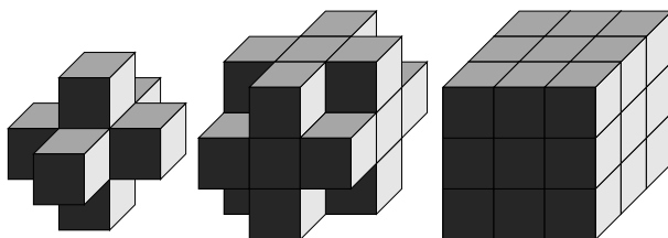
FIGURE 4. Différents voisinage du cube central, 6-voisinage, 18-voisinage et 26-voisinage.
