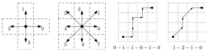
FIGURE 5. Codages de Freeman en 4- et 8-connexité suivis de codages de courbes 4-connexe et 8-connexe.
