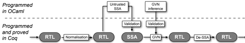
FIGURE 1. Middle-end SSA ajouté au compilateur CompCert, au niveau de la représentation RTL.
